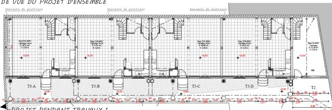
PROJET PENDANT TRAVAUX 1
